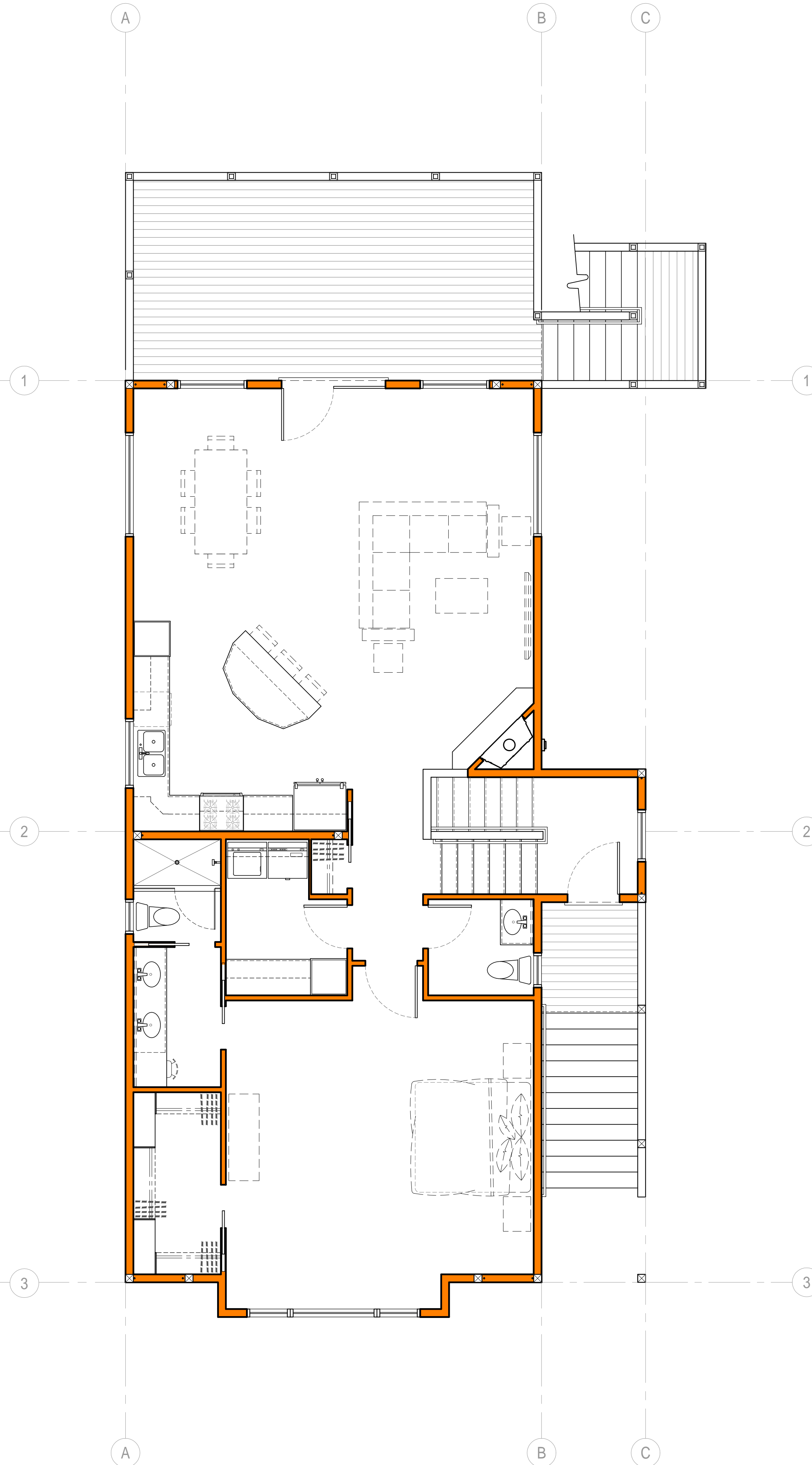
UF UPPER FLOOR
